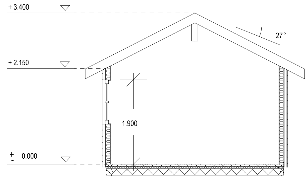
Snitt A-A
